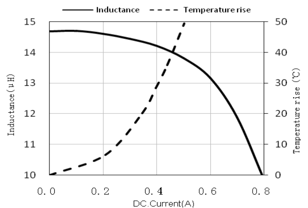
SPH252012H150MT
