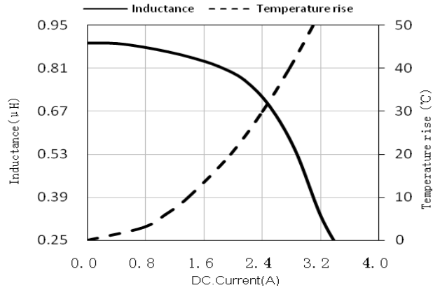
SPH252012H1R0MTY03
