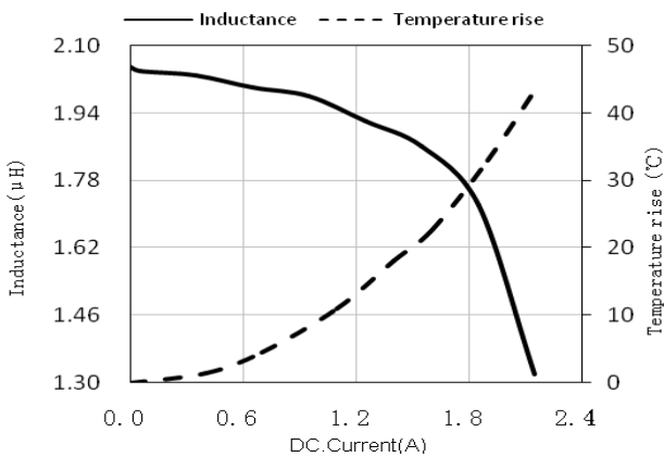
SPH252012H2R2MT
