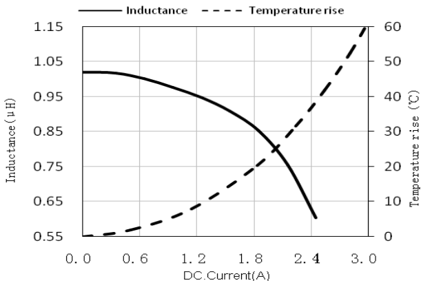
SPH252012H1R0MT
