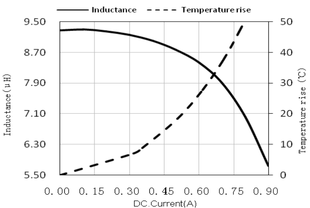
SPH252012H100MT
