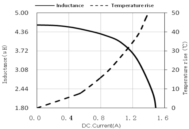
SPH252012H4R7MT
