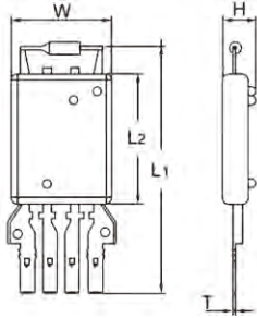
Dimension (尺寸图)
